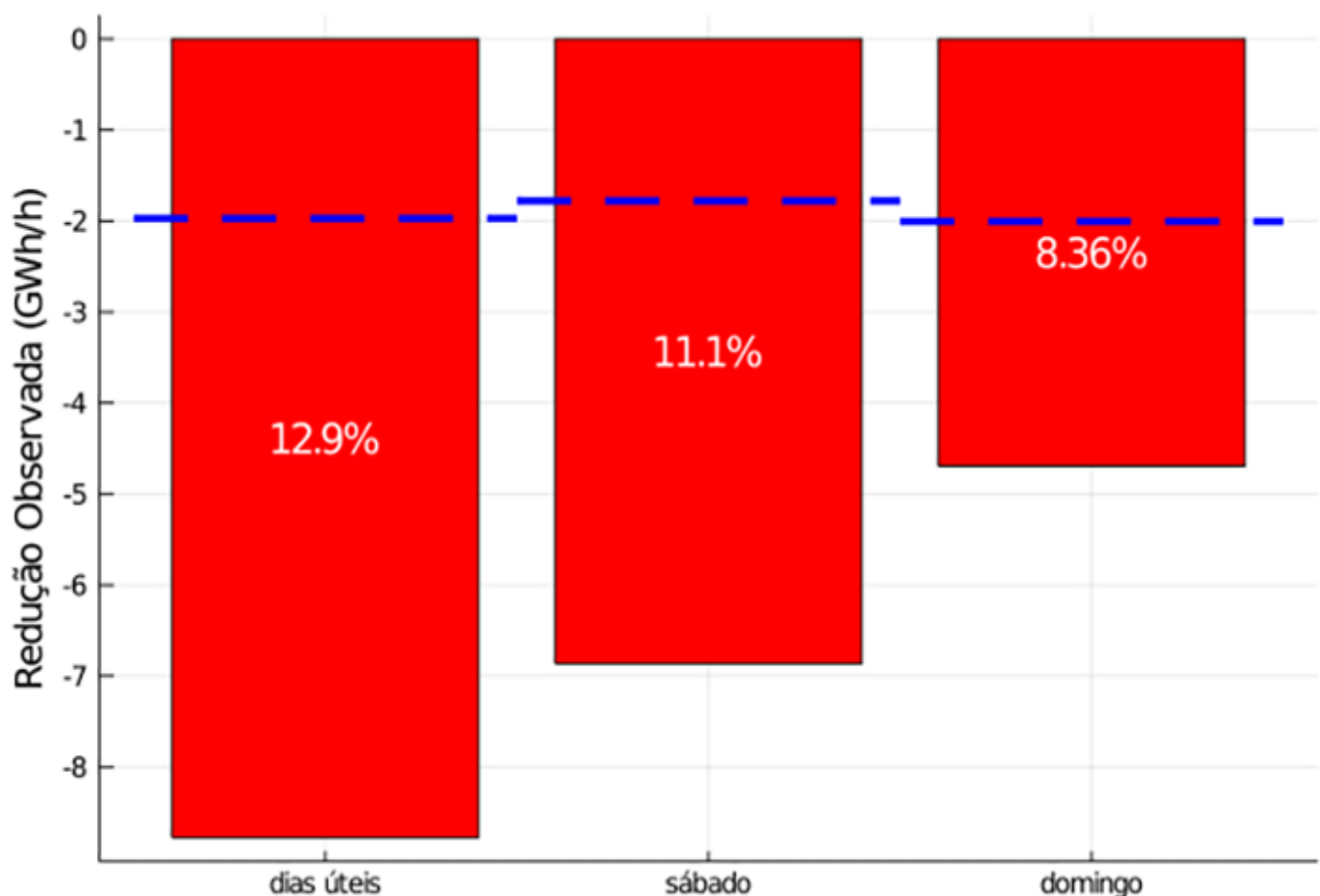
Figura 3 – Reduções observadas (em Gigawatt médio e percentual) para dias úteis e dias de fins de semana com relação ao cenário contrafactual (barras vermelhas) – valores críticos para teste de hipótese (significância 5%) com hipótese nula de que não houve redução
