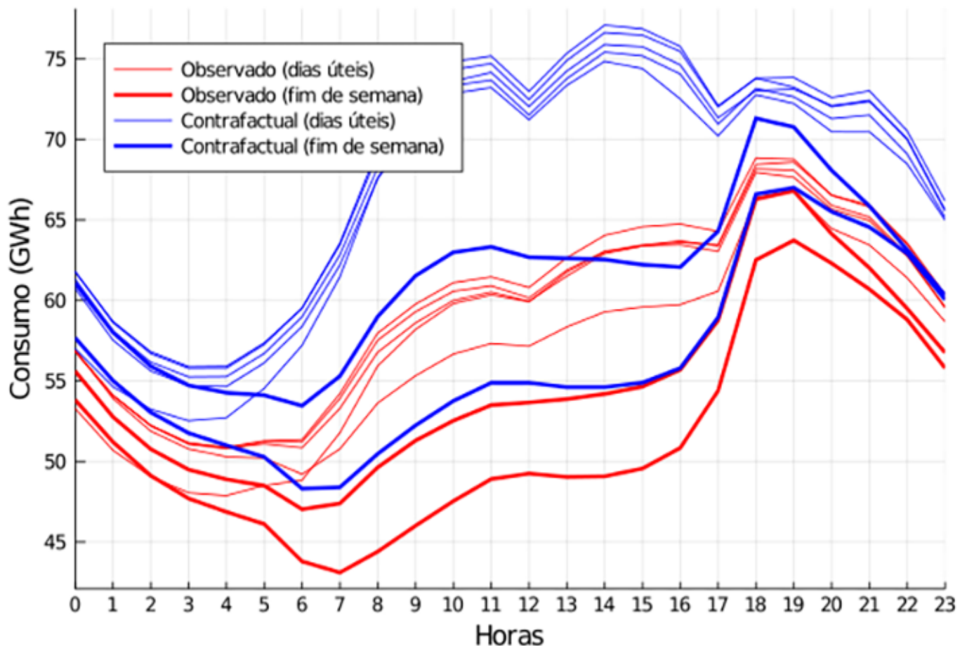
Figura 2 – Curvas de carga para diferentes dias da semana: dias úteis (linhas finas), dias de fins de semana (linhas em negrito) – curvas construídas com base no histórico observado (linha vermelhas), curvas construídas utilizando o cenário contrafactual (linhas azuis)
