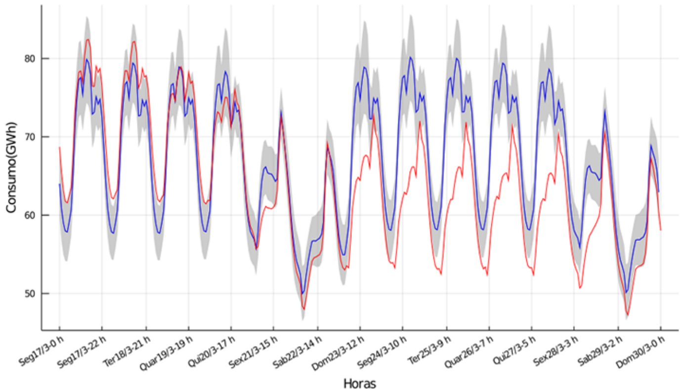
Figura 1 – Sequência de suas semanas após intervenção (de segunda, 0h do dia 17 de março de 2020, a domingo, 23h do dia 30 de março de 2020): histórico observado (linha vermelha), cenário contrafactual (linha azul), faixa de 95% de confiança para o cenário contrafactual (área cinza)
